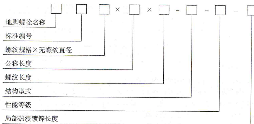
图 7 产品完整标记
