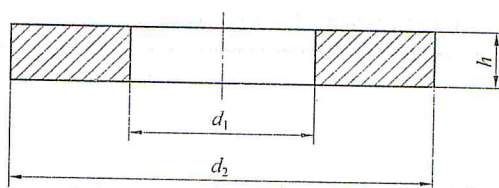
图 B.1 平垫圈的型式
