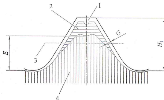
1—全脱碳；2—不完全脱碳；3—中径线；4—基体金属
