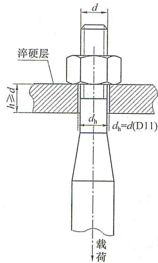
图 14 轴向拉伸试验
