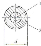
1—试件轴心线；2— 1/2 半径区域
