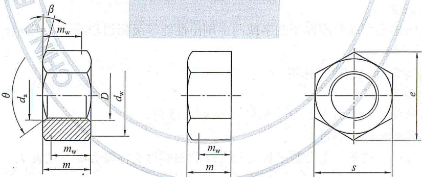
图 6 螺母型式
