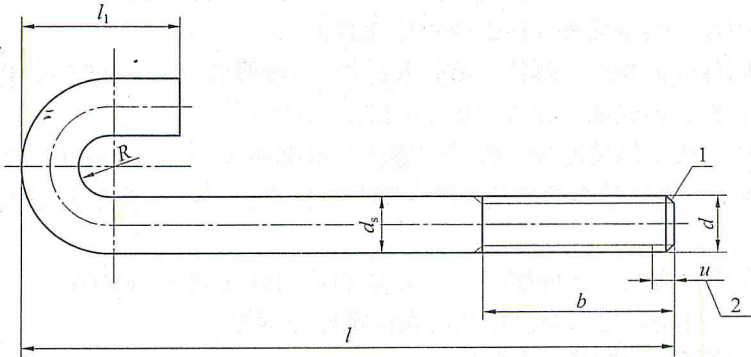
1—末端应倒角，按 GB/T 2 规定；2—末端不完整的螺纹长度 u \leq 2P
