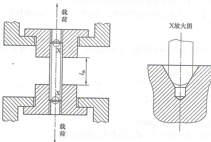
图10 保证载荷试验
