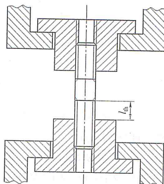
l_{th} —试验夹具中地脚螺栓未旋合螺纹的长度
