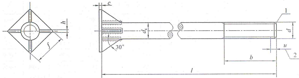
图 4 T 型地脚螺栓型式
