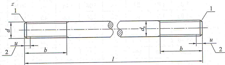
图 5 双头型地脚螺栓型式
