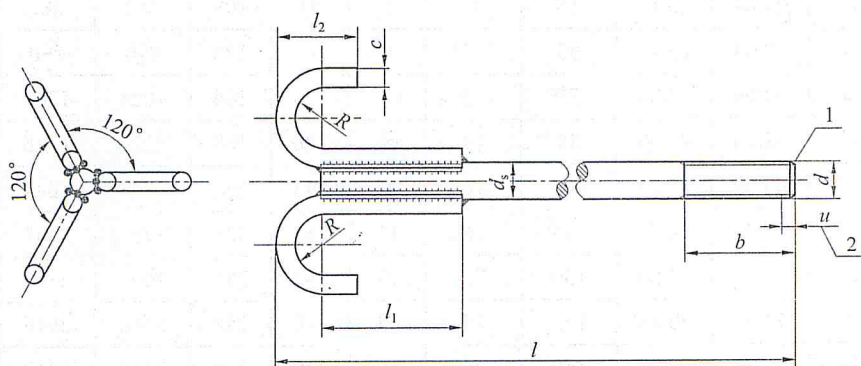
图3 棘爪型地脚螺栓型式
