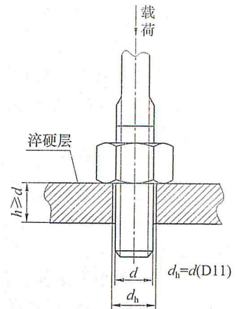
图 15 轴向压缩试验
